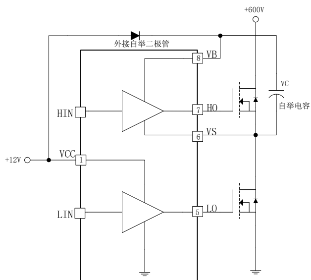
图 8-3. EG2108D 自举电路结构
