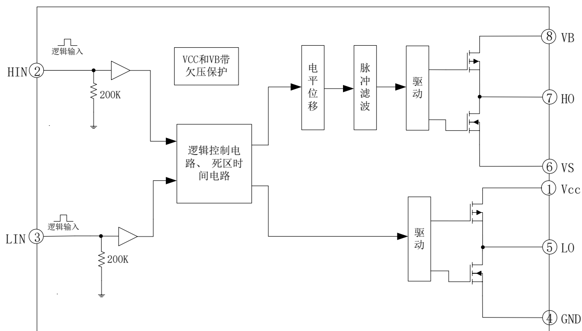
图 5-1. EG2108D 内部电路图
