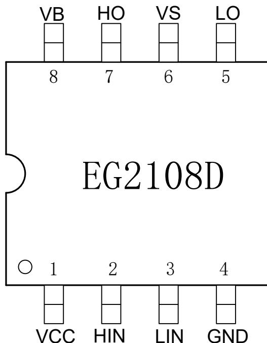
图 4-1. EG2108D 管脚定义
