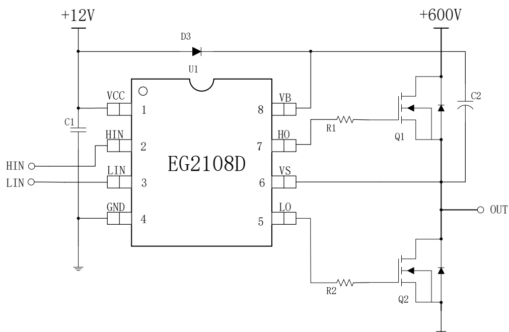
图 6-1. EG2108D 典型应用电路图
